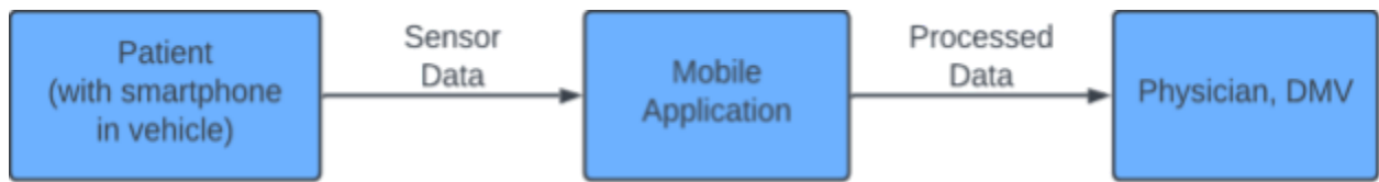
DFD Level 0
