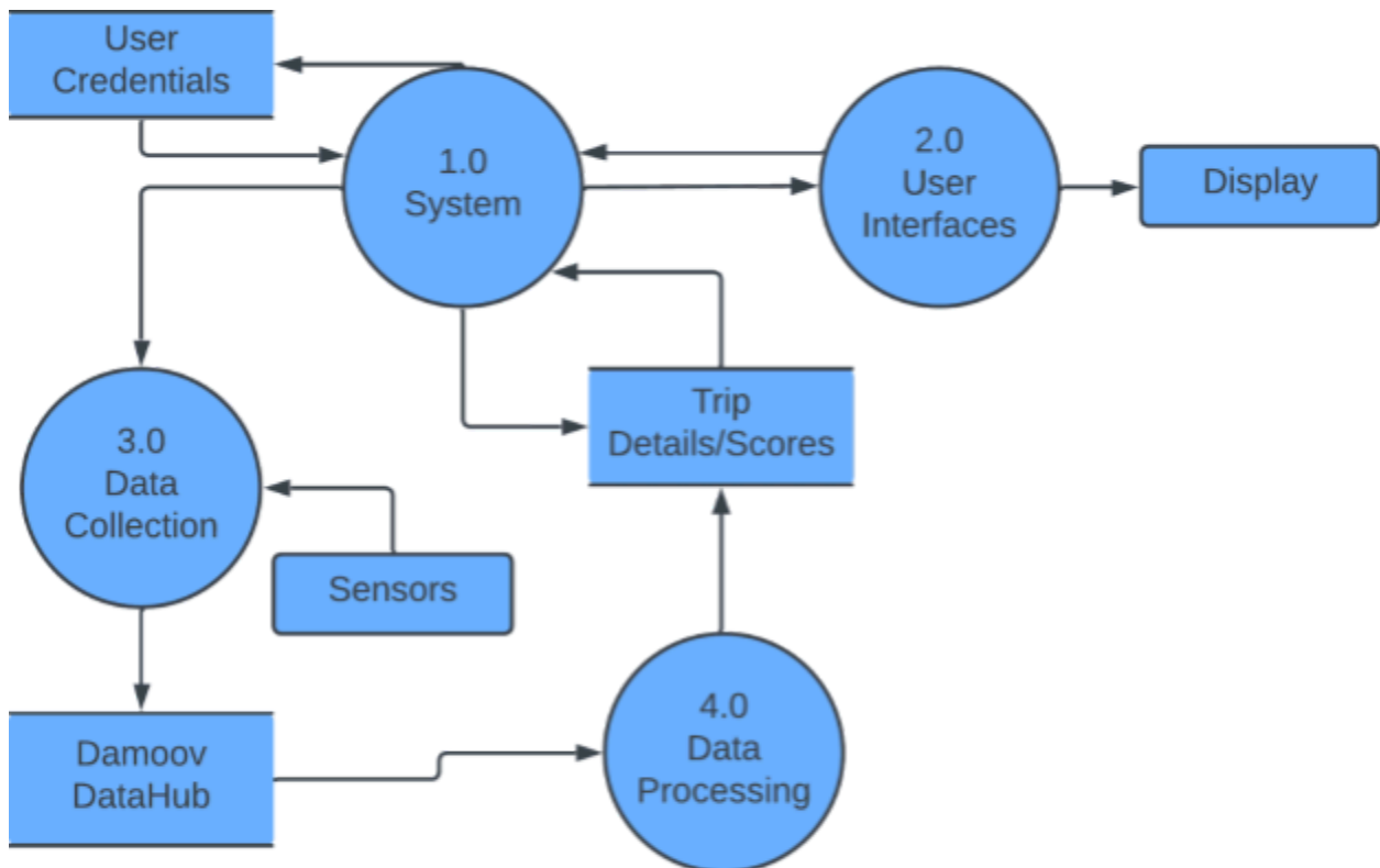
DFD Level 1
