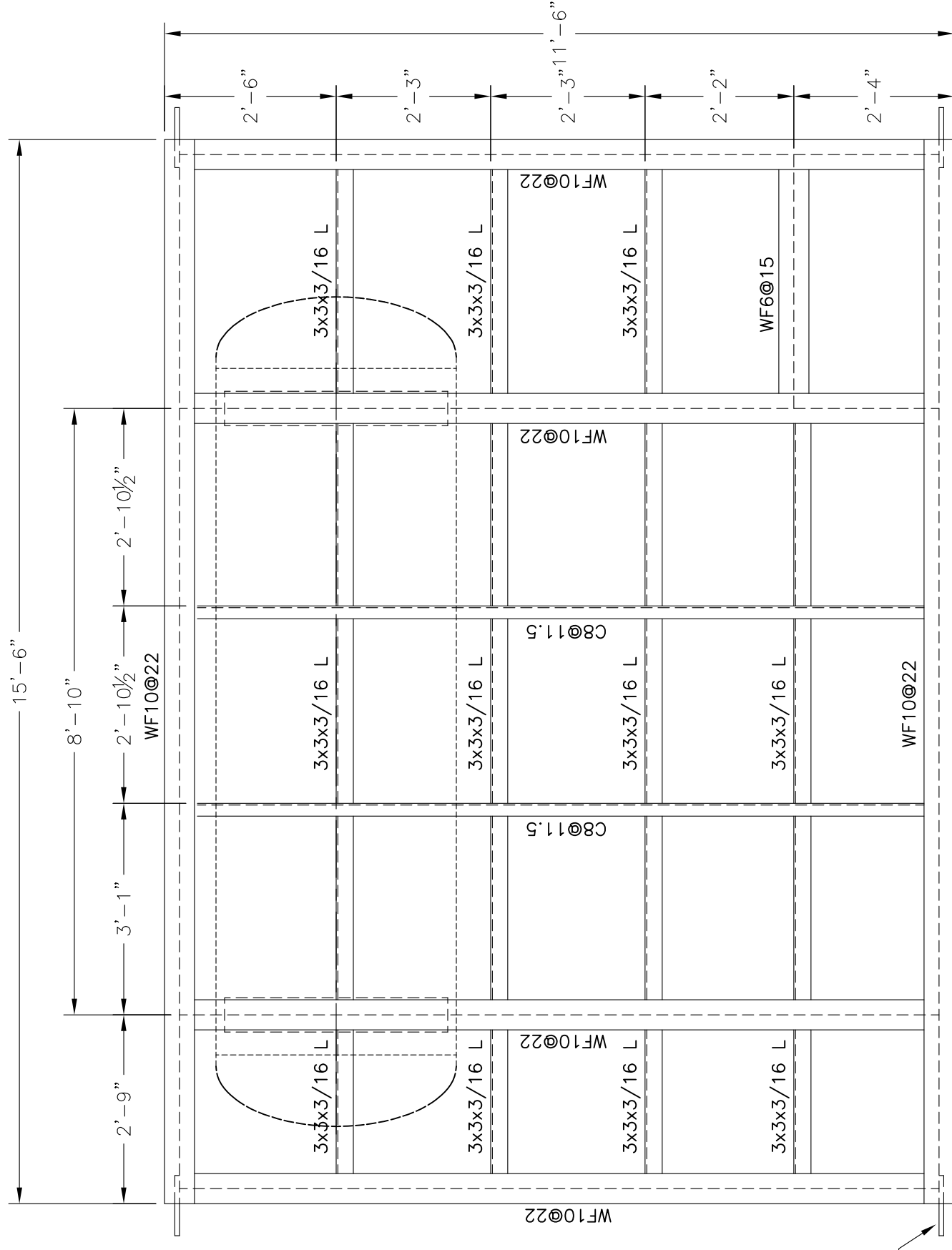
SKID LAYOUT SCALE: 1'-0" = 1/2"
