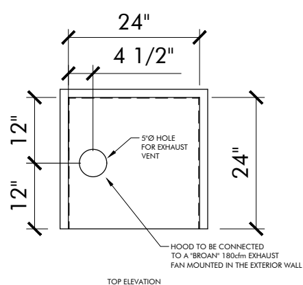
TOP ELEVATION
