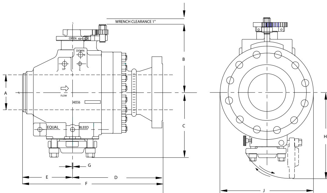
FLANGEWELD TYPE
