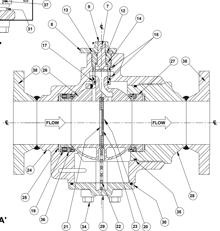
SECTION 'B-B'
