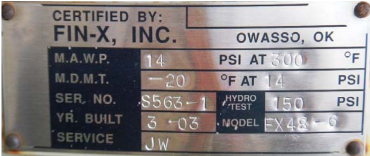
EJW COOLER
